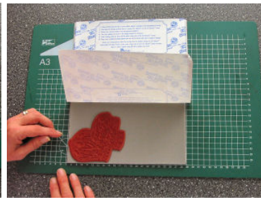
Plak de stempel met de achterkant op de EZ mount.
